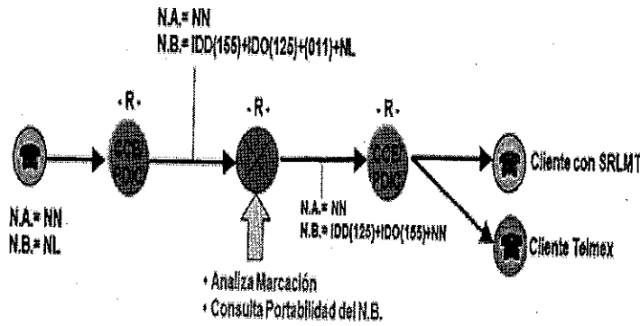
DIAGRAMA DE ENTREGA DE LLAMADA TELMEX(125) → AXTEL(155) → TELMEX(125)
